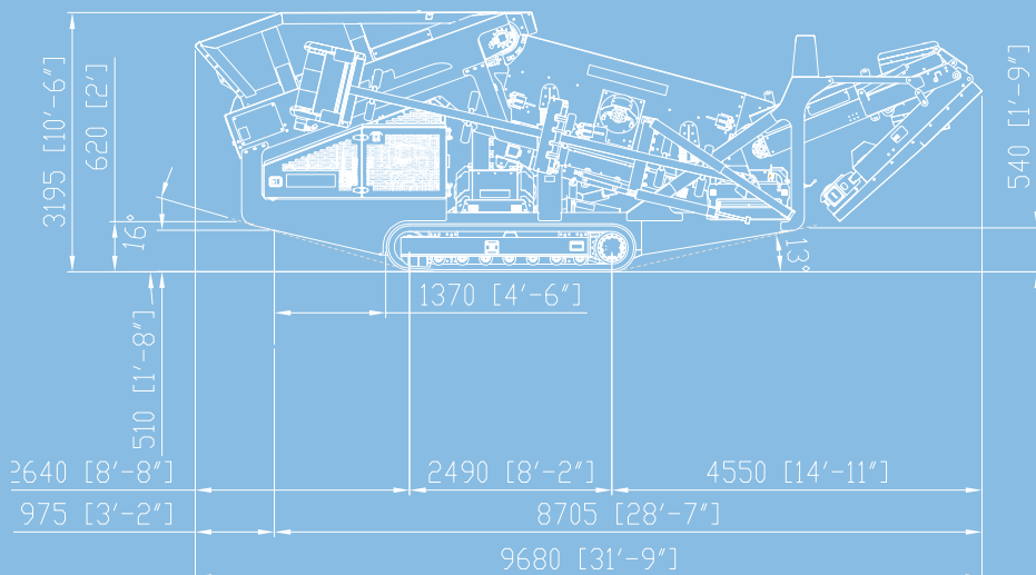
Схема MS 12 Z-AD в транспортном положении
