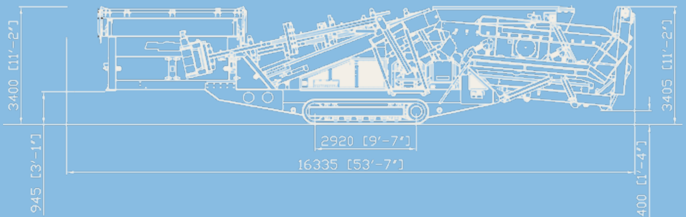
Seitenansicht MS 16 Z Transportstellung
