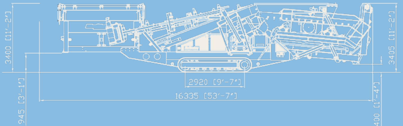
Vista lateral M 16 Z en posición de transporte
