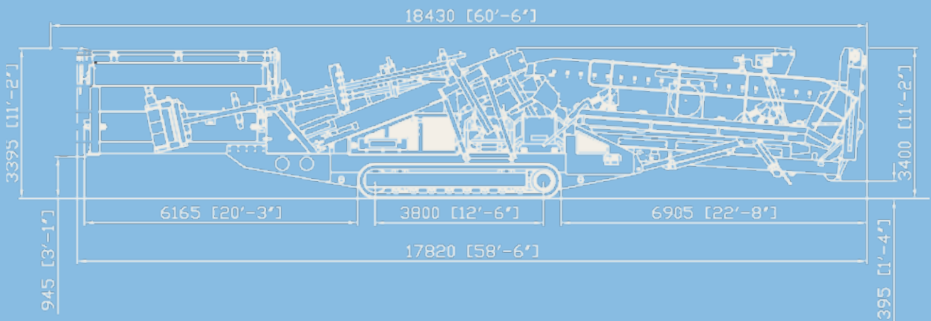
Vista lateral MS 19 Z en posición de transporte
